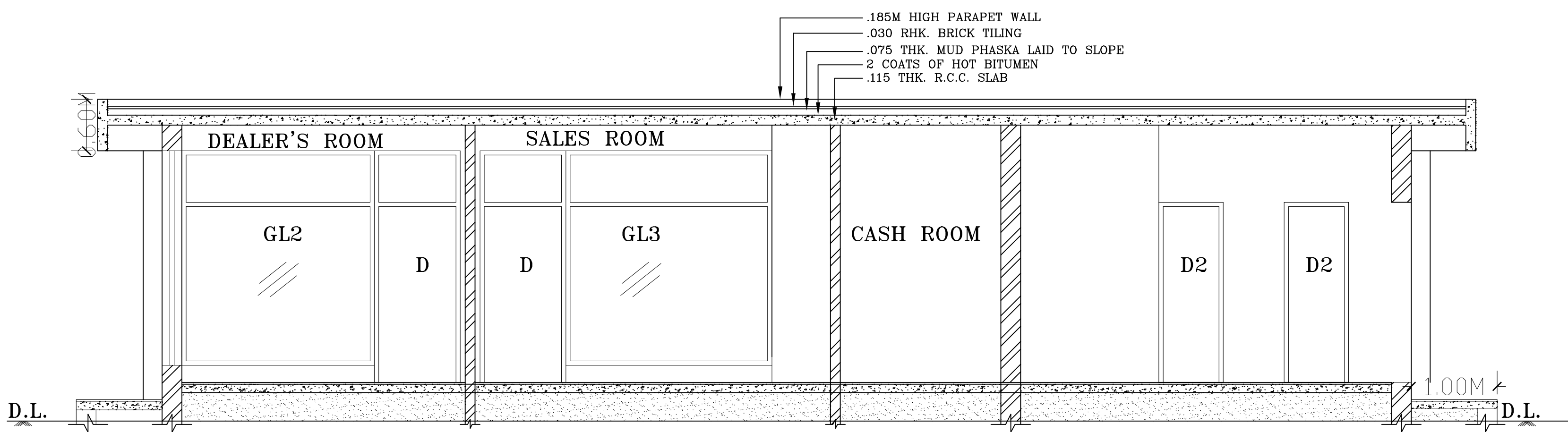
SECTION A-A
