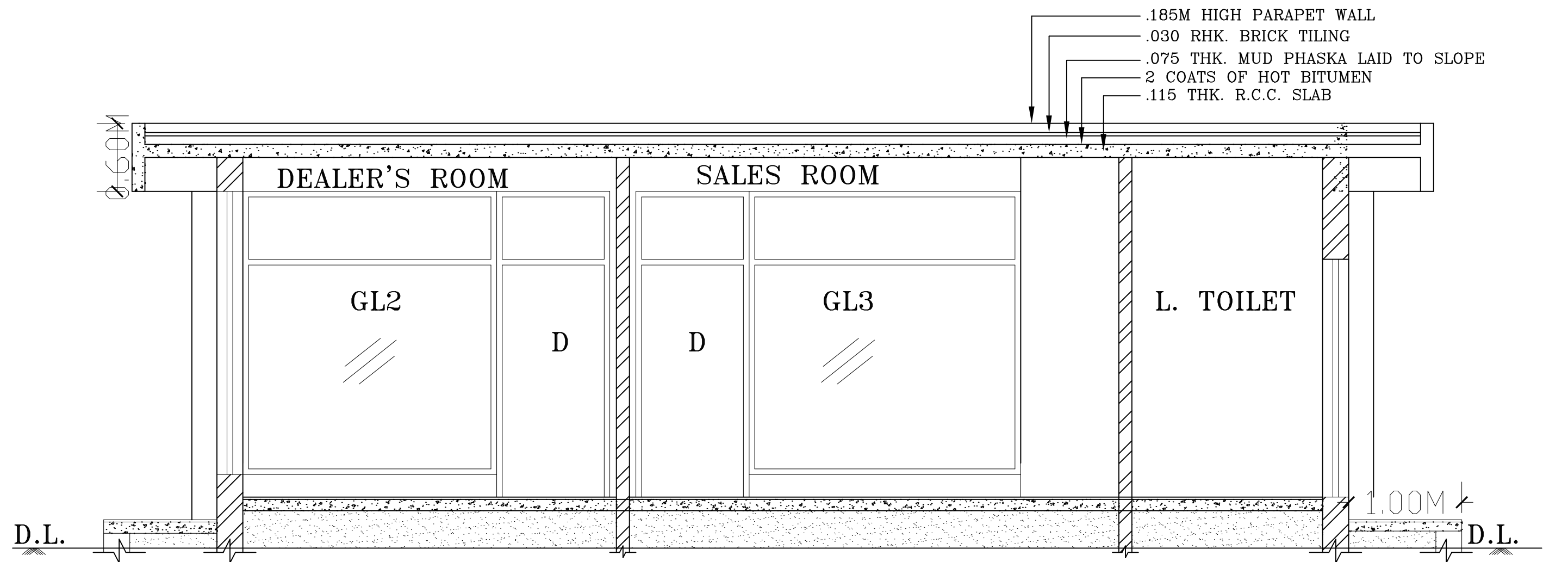
SECTION A-A
