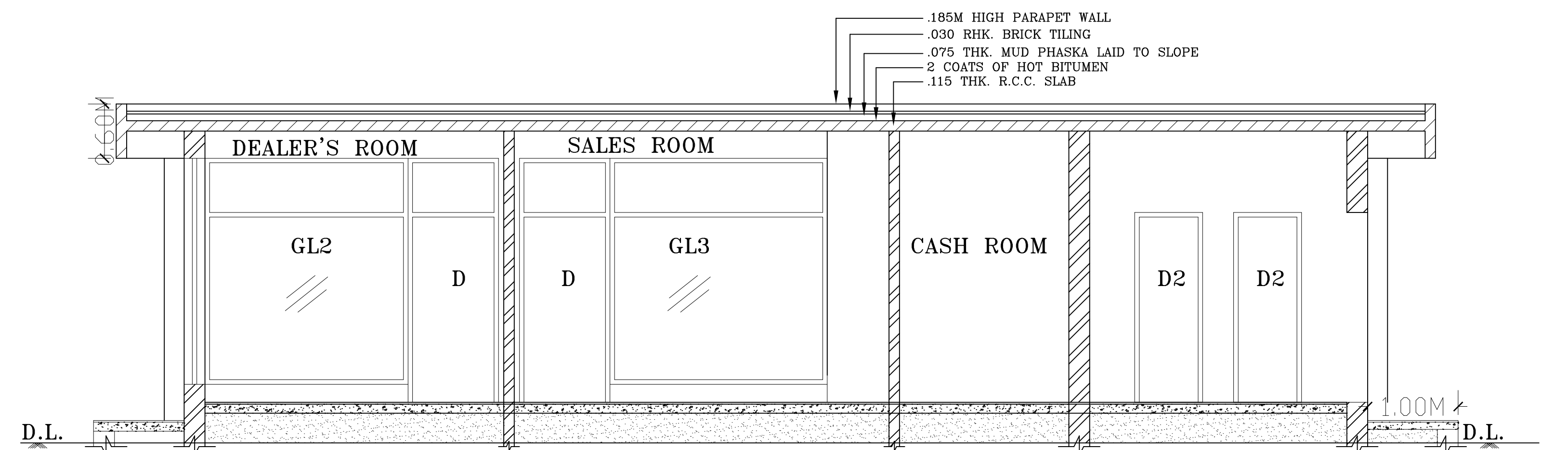
SECTION A-A
