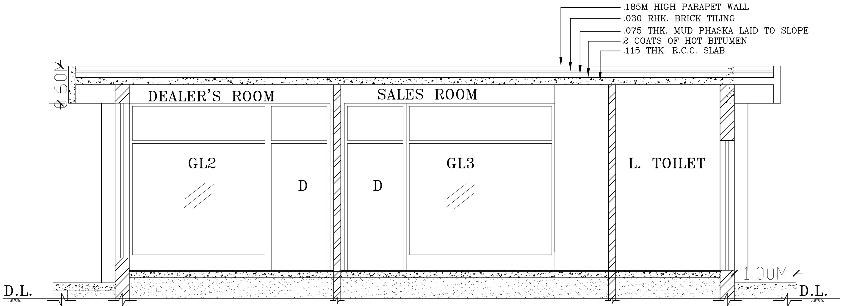
SECTION A-A
